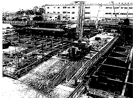
(写真1) 免震基礎工事
